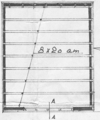
PLAT BALKLAAC
