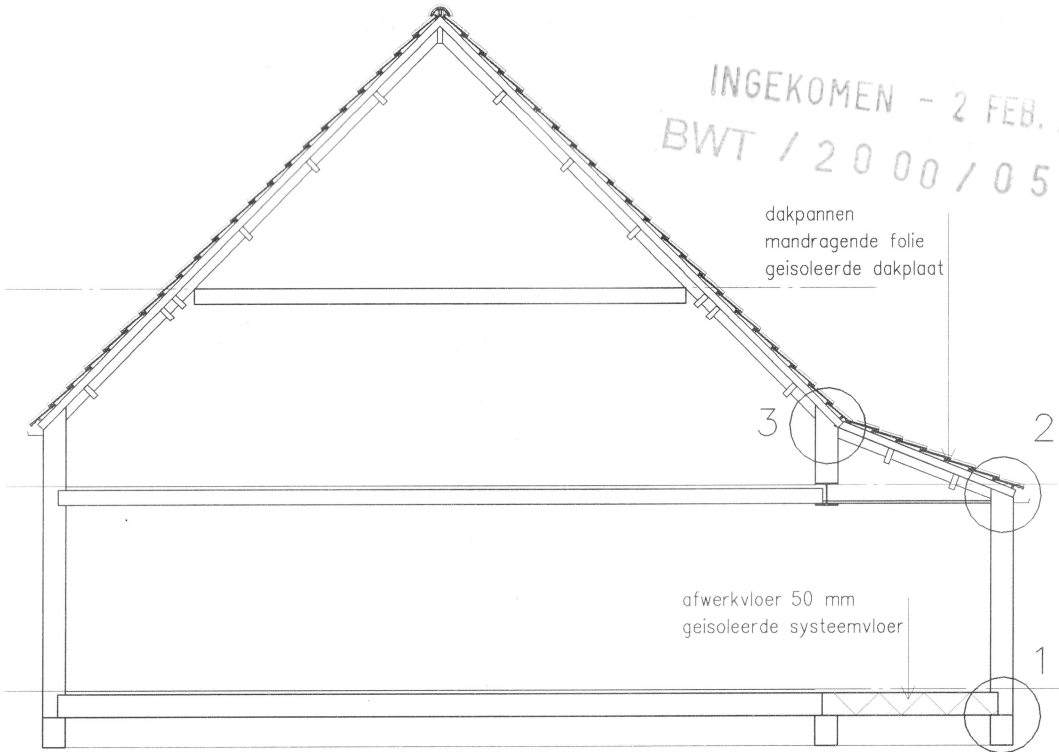
doorsnede nieuw
