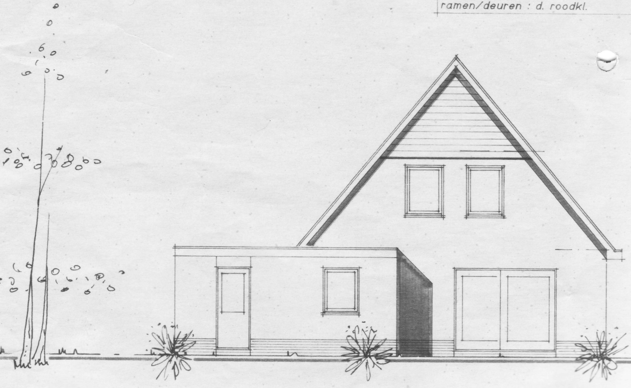
achtergevel
